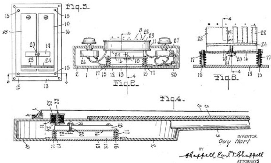
Snímač z patentu 2,087,106
